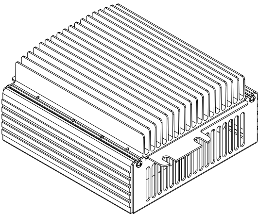
Figure 32 Ребра TCM
