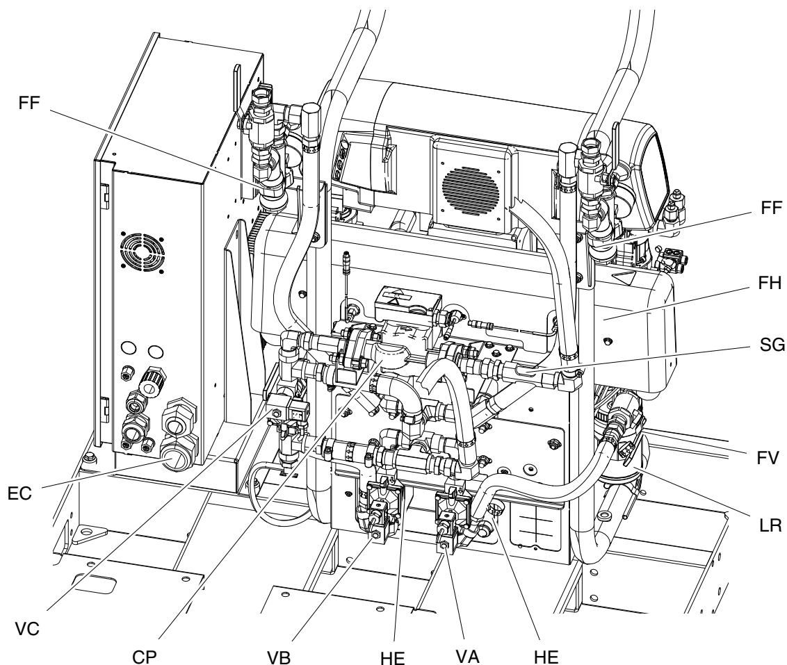
Figure 4 Вид сзади
